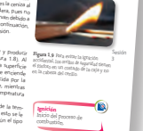
Figura 1.9 Una cerilla encendida produce un cambio en la temperatura del entorno y en la materia que interactúa con él.
