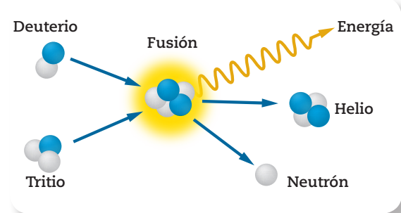
Figura 1.55 El proceso de fusión entre el deuterio y el tritio produce un núcleo de helio, un neutrón y una gran cantidad de energía.
