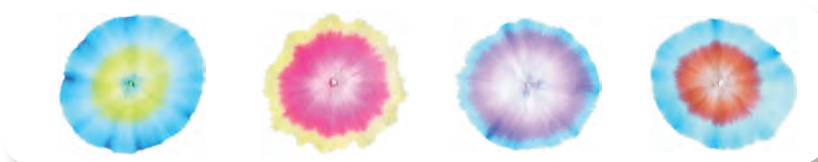
Figura 1.32 Las tintas de diferentes colores son mezclas de pigmentos con un líquido que puede ser agua o alcohol.
