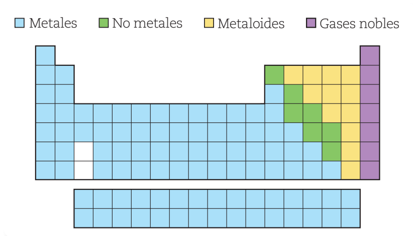
Figura 2.42 Clasificación de los elementos basada en sus propiedades.
