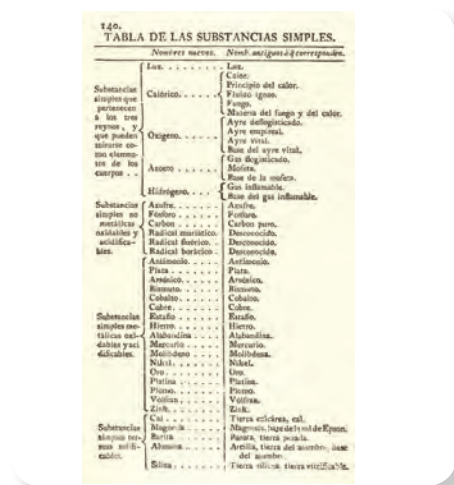
Figura 2.38 Tabla de organización de sustancias elementales de Lavoisier en su libro Tratado de Química Elemental de 1789.
