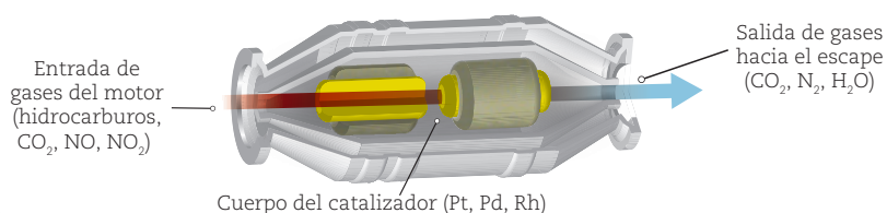
Figura 2.28 Partes de un convertidor catalítico y los elementos químicos que catalizan las reacciones en su interior.
