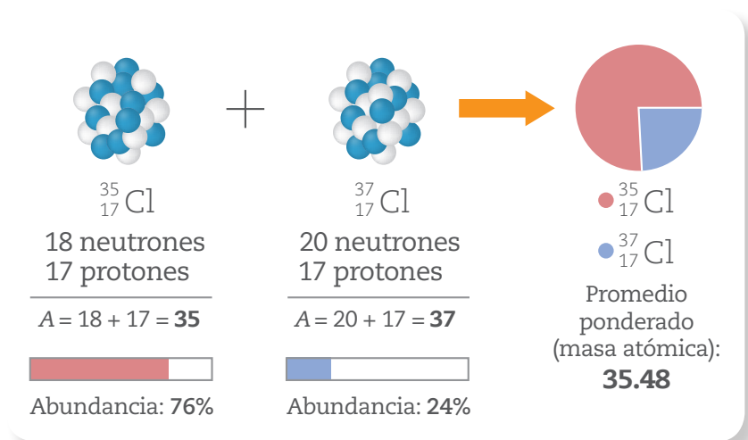
Figura 2.43 Isótopos del cloro y cálculo de su masa atómica.
