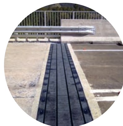
Figura 1.80 Para evitar que algunos puentes se deformen o se rompan, se colocan separaciones entre los bloques que los conforman.
