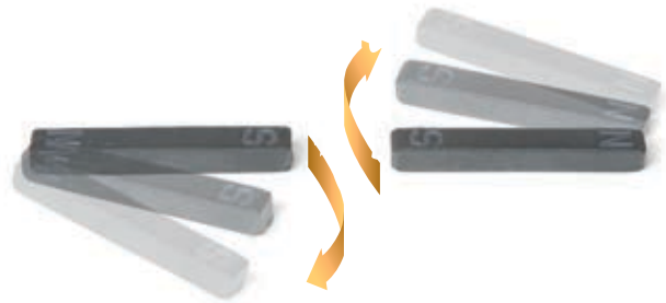
Al aproximar polos iguales de los imanes de barra, éstos se repelen o rechazan.
