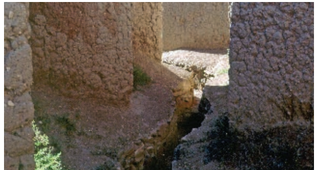
Sistema de drenaje en Paquimé.
